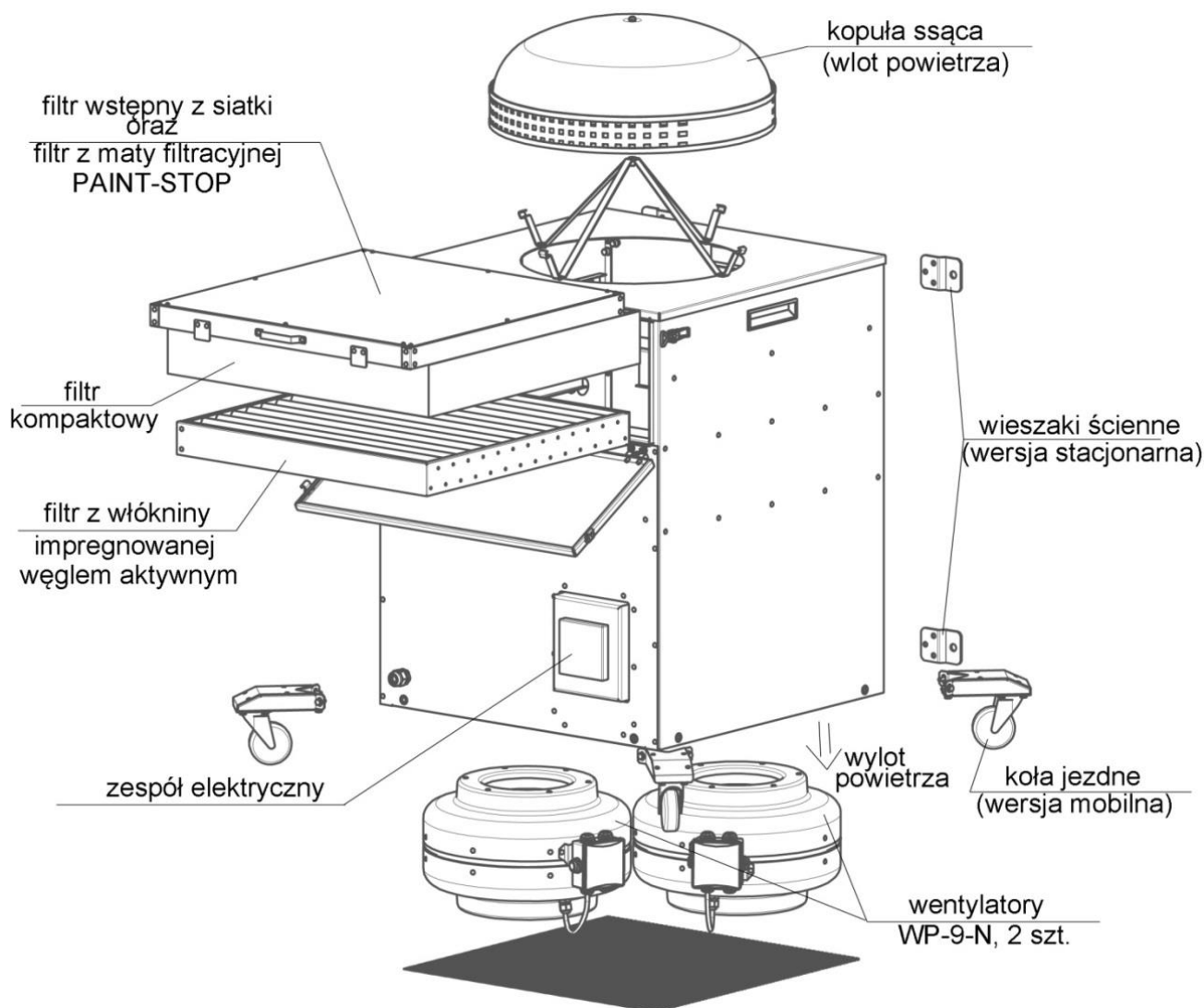
Rys. 2 Budowa urządzenia typu RAK-2000-RC
